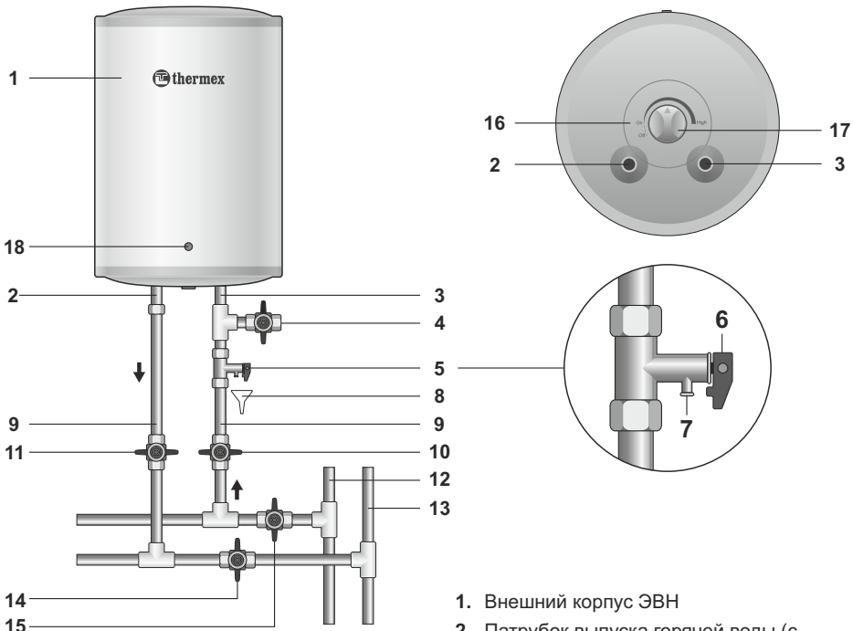
Рис. 1 Схема подключения и элементы управления.
